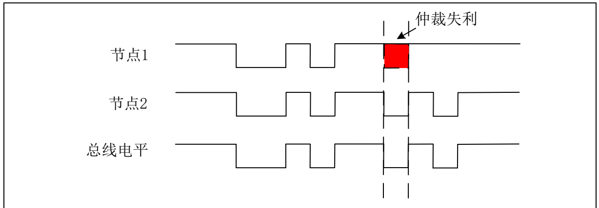
图 7 仲裁机制
