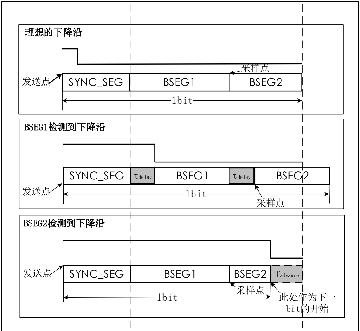
图 6 重同步跳跃
