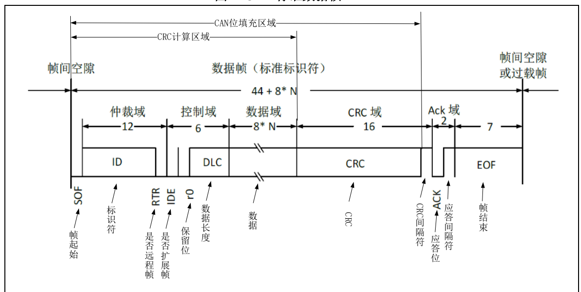
图 4 CAN 标准数据帧
