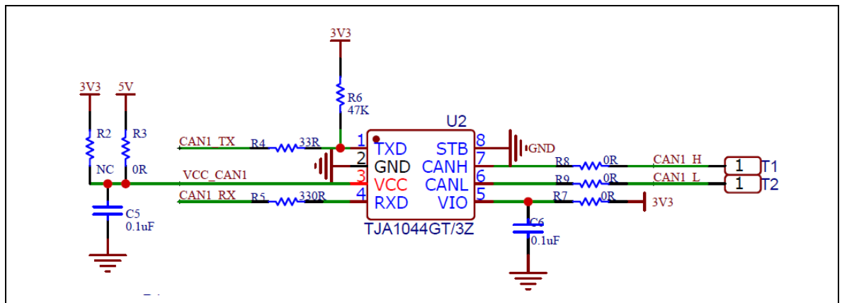
图 18 CAN 电平转换器硬件设计
