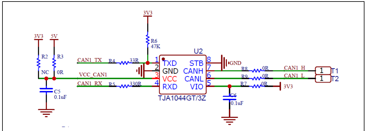
图 17 CAN 电平转换器硬件设计
